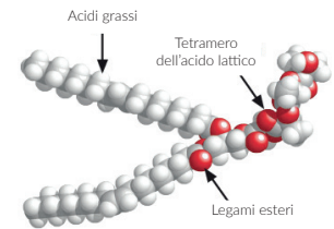
FIGURA 1: STRUTTURA MOLECOLARE DEL 3-D MICROEMULSION
